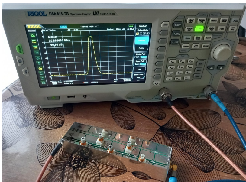
Filtre de sortie 37Mhz home made
