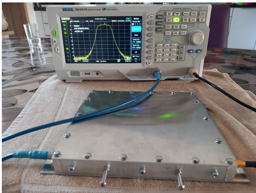
Filtre d'entrée 437 MHz home made
